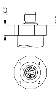
M12x1 (4 конт.) (IP 67)
