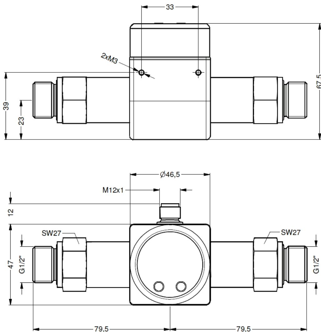
Рисунок Б.1 – Габаритные размеры корпуса прибора
