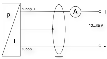
2-проводное исполнение: 4...20 мА
