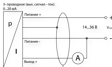
3-проводное исполнение: 0...20 мА
