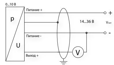
3-проводное исполнение: 0...10 В
