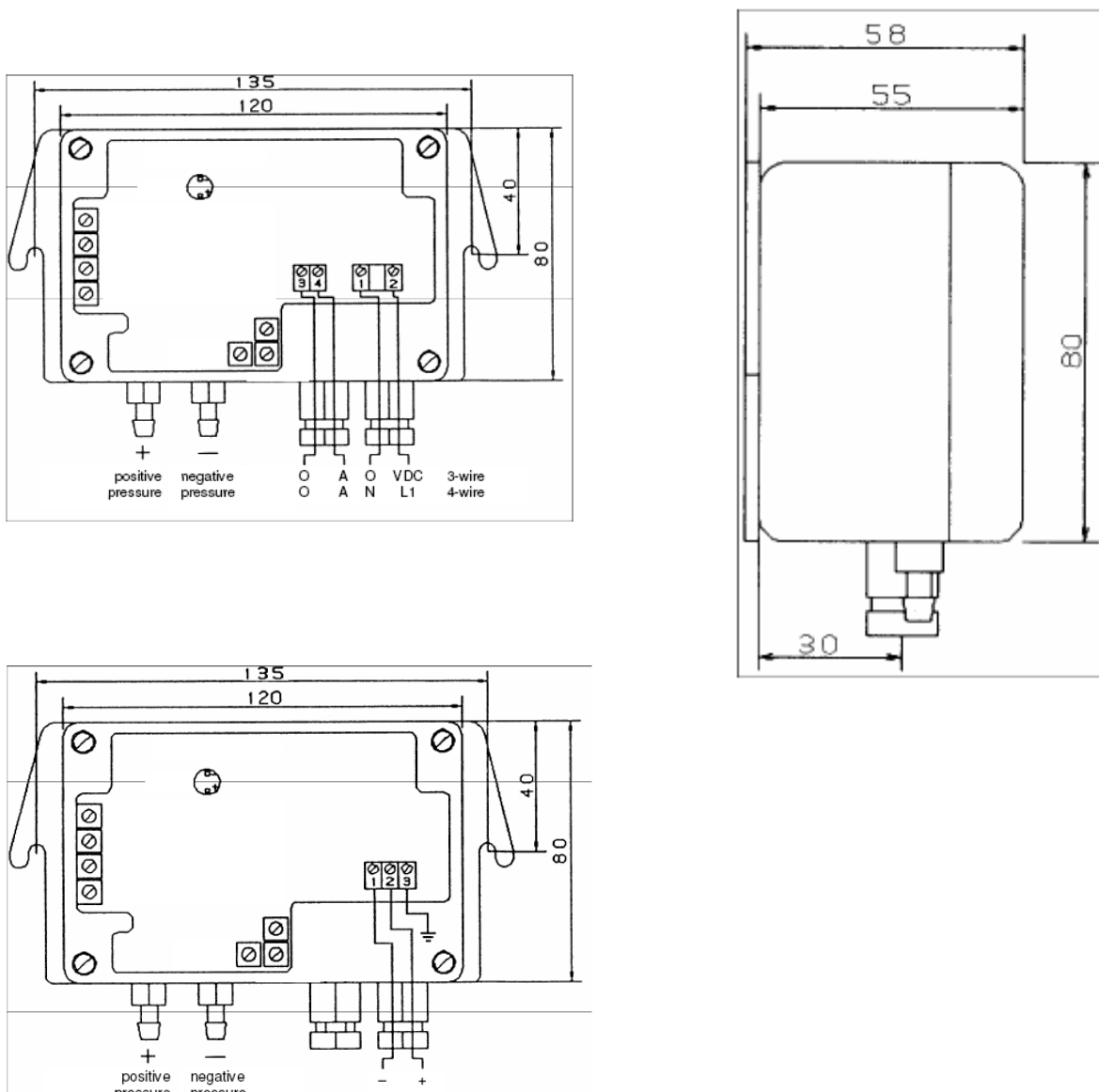
Рисунок Б.1 – Габаритные размеры датчика DPS 100
