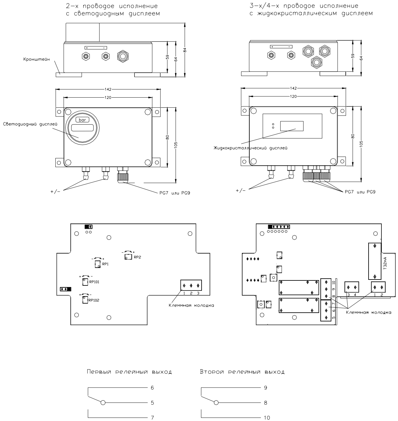
Рисунок Б.2 – Габаритные размеры датчика DPS +
